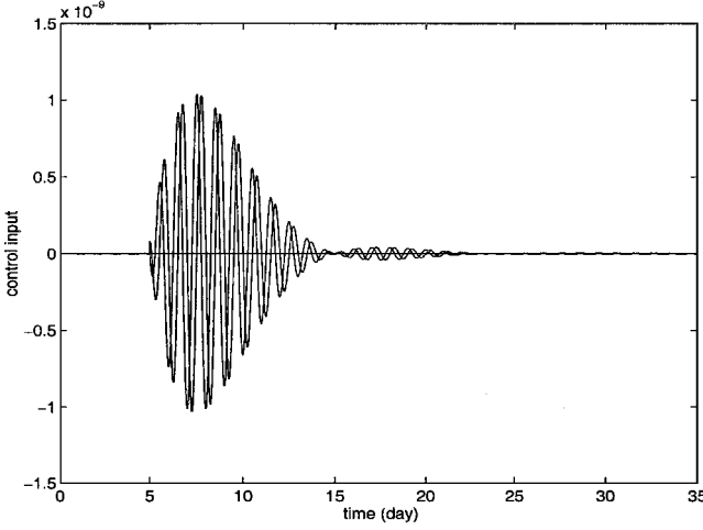
Fig. 5 Control input.
